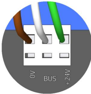
0V - colore MARRONE BUS - colore BIANCO 24V - colore VERDE
